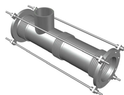
Compensatore a spinta bilanciata universale
