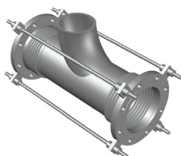
Compensatore a spinta bilanciata
